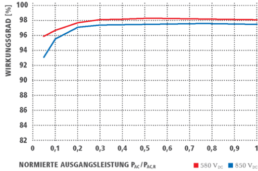
WIRKUNGSGRADKURVE FRONIUS ECO 27.0-3-S
