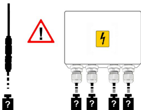
Ryc. 13: Złącza DC i skrzynki połączeniowe modułów z dławikami PG - zintegrowane przepusty absorbują siły tylko w ograniczonym zakresie.
