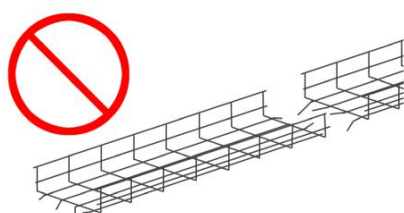
Ryc. 5: Kratka kablowa z wolnymi końcami prętów i ostrymi krawędziami. Uwaga – niebezpieczeństwo uszkodzenia izolacji!
