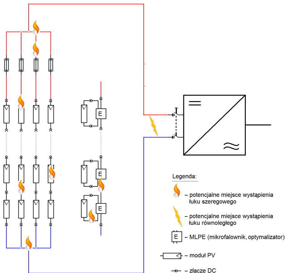
Ryc. 1. Potencjalne miejsca wystąpienia łuków szeregowych i równoległych w instalacjach PV.
