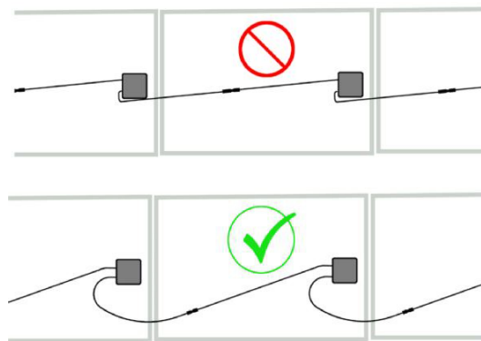
Ryc. 11: W przypadku modułów montowanych poprzecznie należy zwrócić uwagę na odpowiednie długości kabli, aby zachować zgodność z promieniem gięcia i uniknąć dodatkowych obciążeń rozciągających na modułowym gnieździe połączeniowym.
