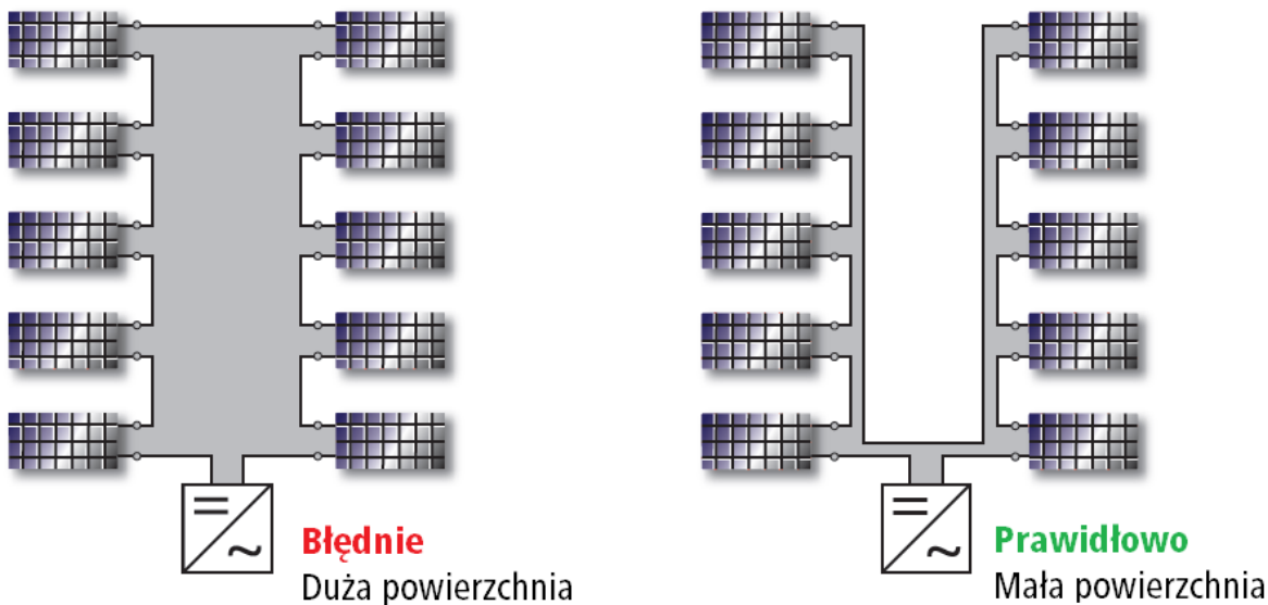
Ryc. 15. Przy układaniu przewodów należy minimalizować powierzchnię pętli.
