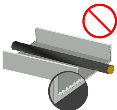
Ryc. 2: Koryta z zadziorami. Uwaga – niebezpieczeństwo uszkodzenia izolacji!
