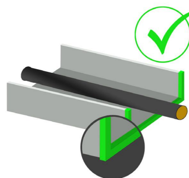
Ryc. 4: Należy stosować ochronę krawędzi lub dodatkowo zabezpieczoną instalację w plastikowych rurach w obszarze krawędzi i ugięć przewodów
