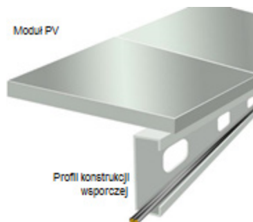
Ryc. 7: Zalecana jest prowadnica kabla zintegrowana w konstrukcji wsporczej
